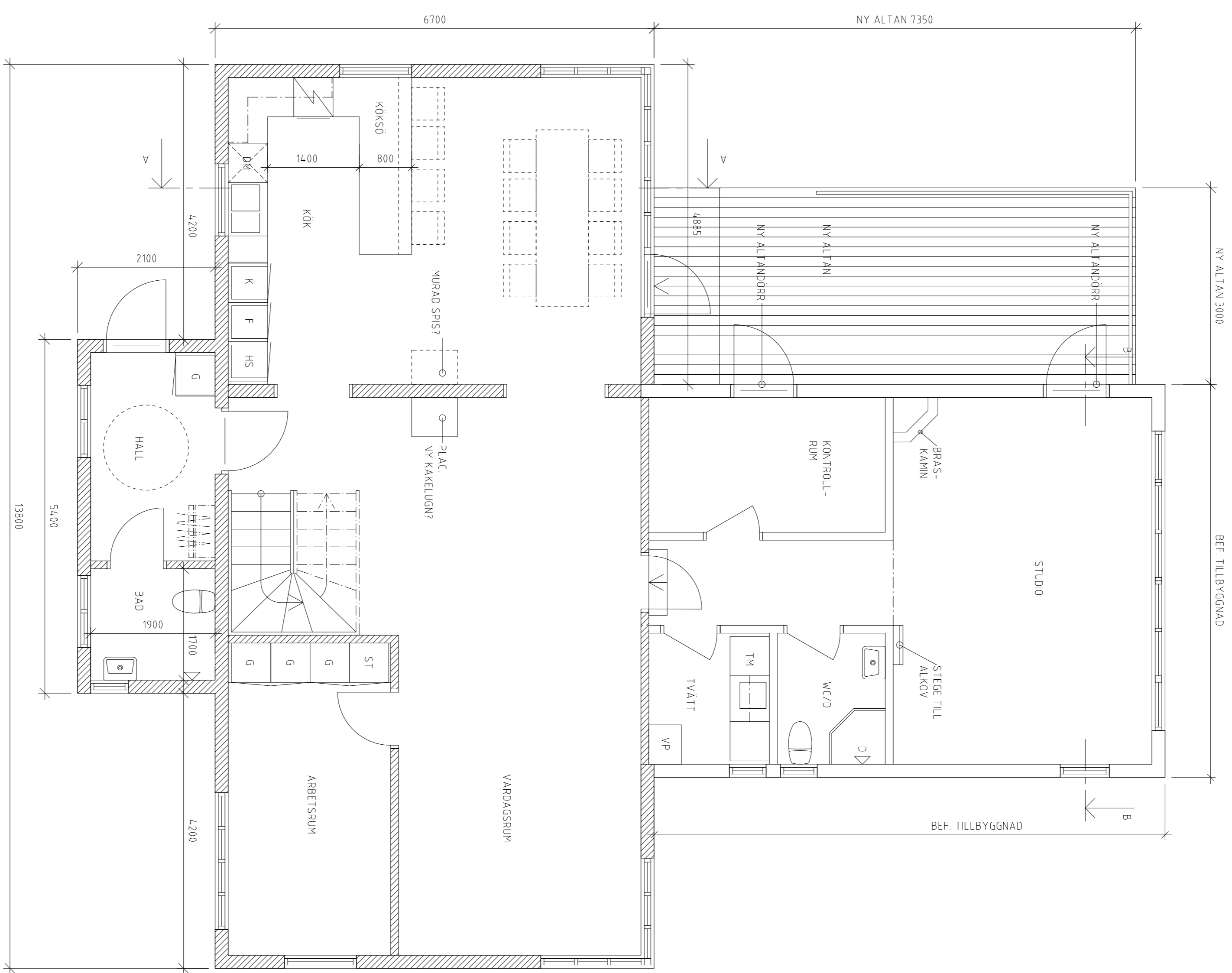
PLAN 1, ENTRÉPLAN
